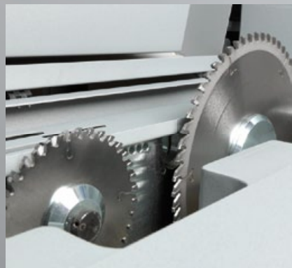
Carro de sierra con agregado principal e incisor
